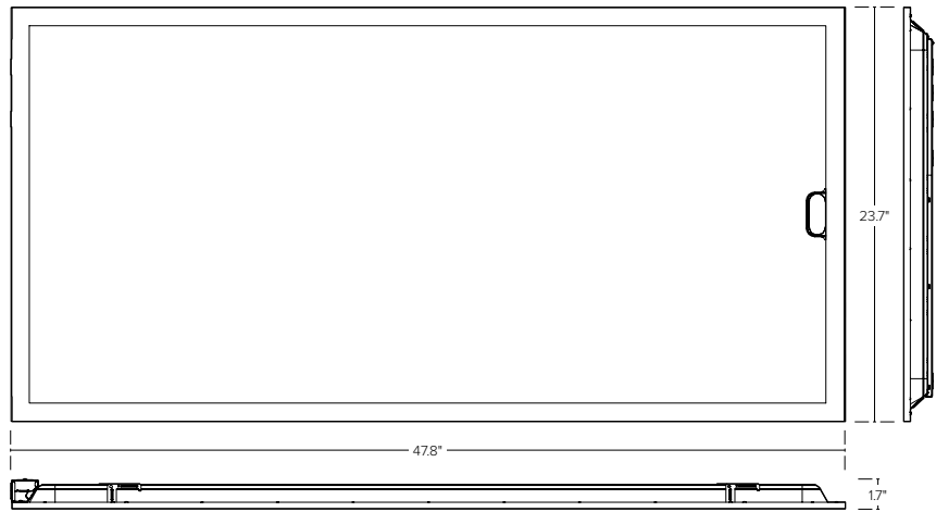
2x4 ESL-ISS-620-24-2040W-3550K
