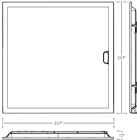
2x2 ESL-ISS-620-22-1525W-3550K
